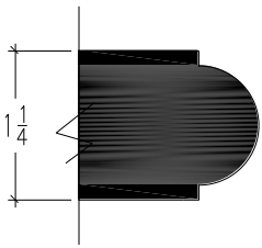
Detail Code Bead (BD)
